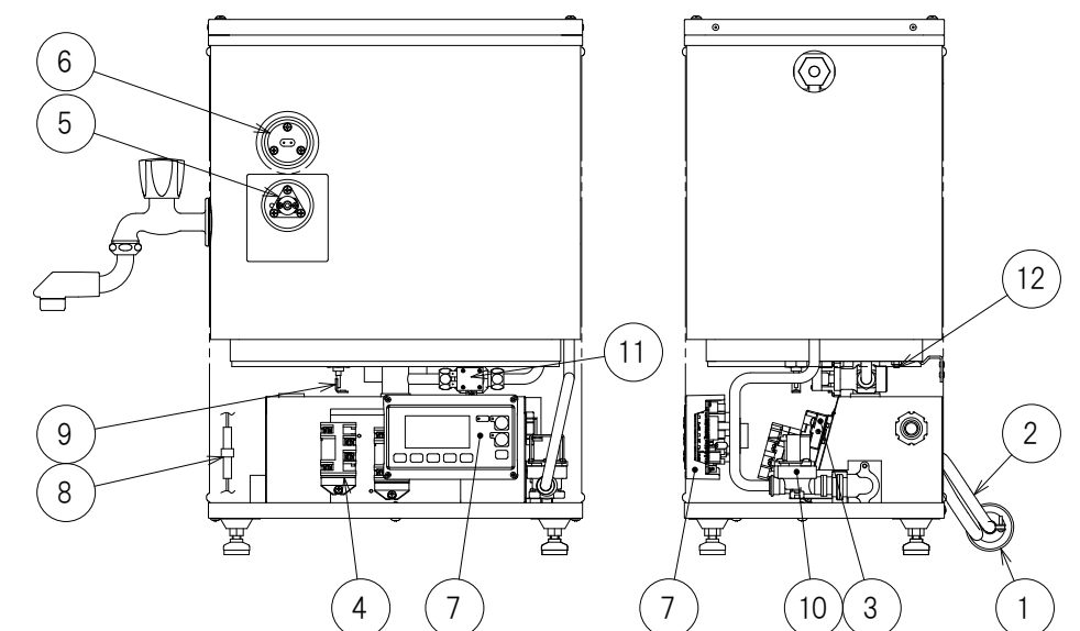
正面図
