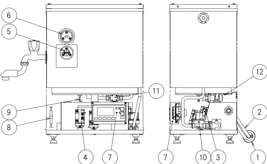
部品配置図 (図はETR12CJL)
