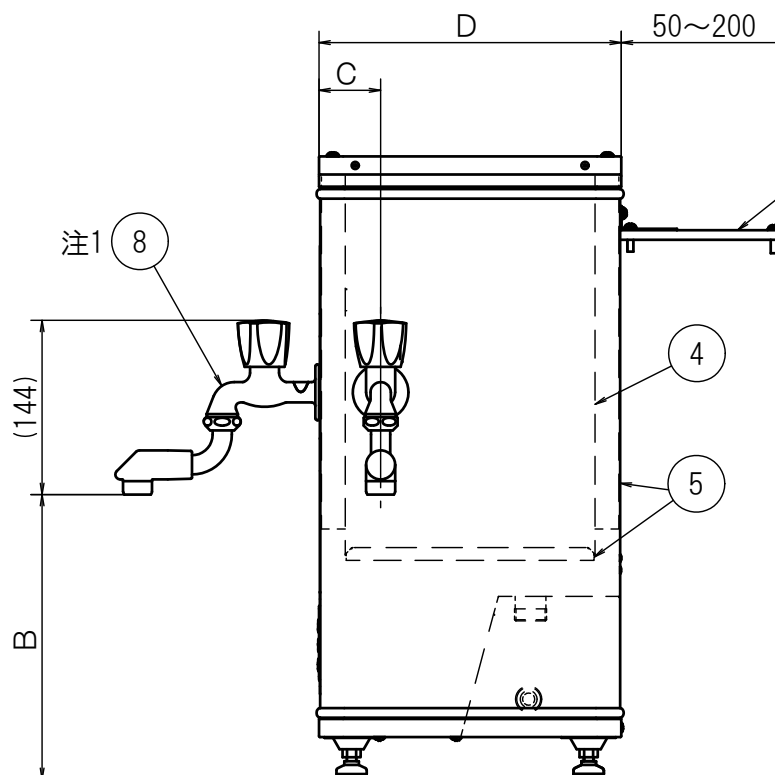
右側面図
