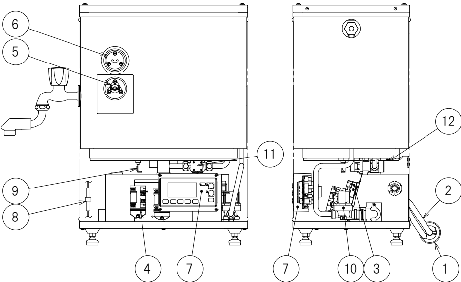
正面図
