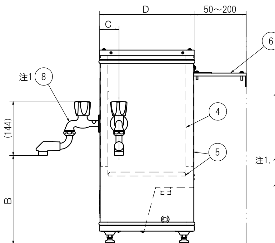
右側面図
