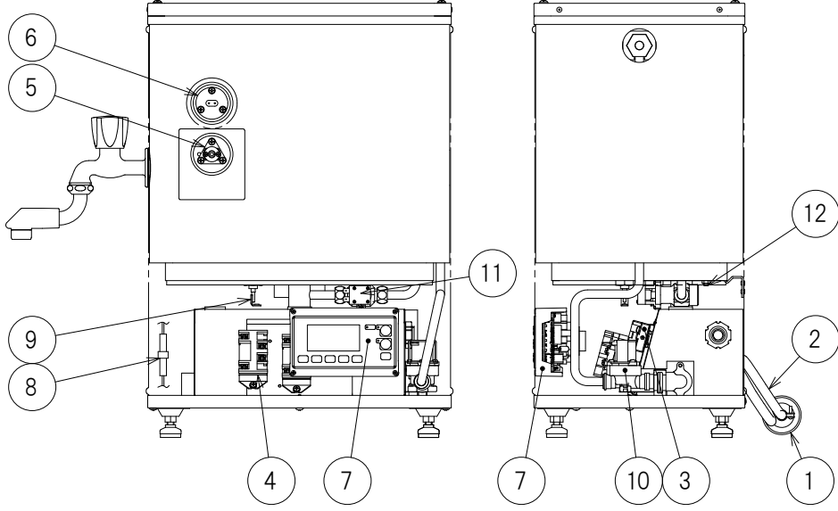
正面図
