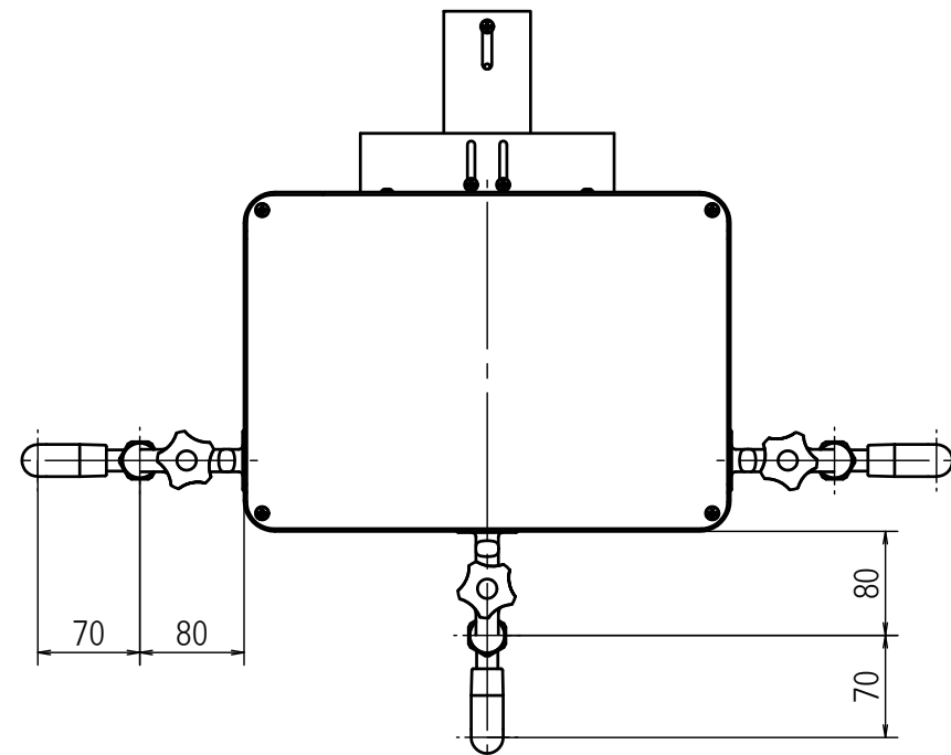
平面図
