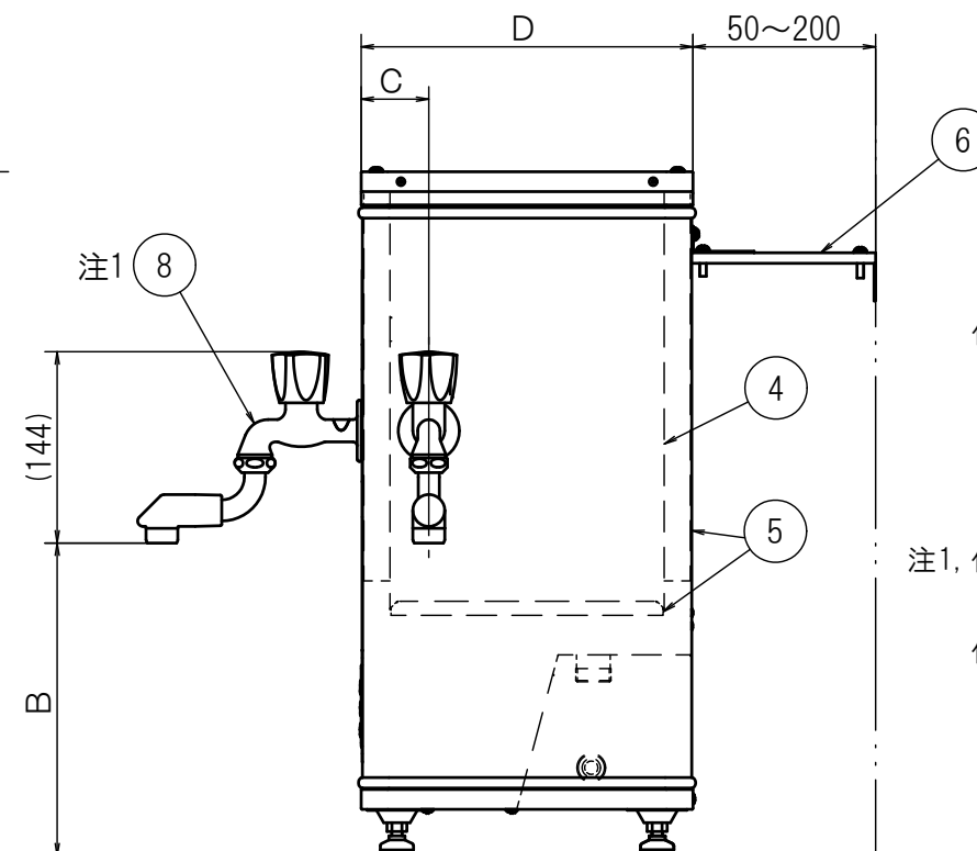
右側面図
