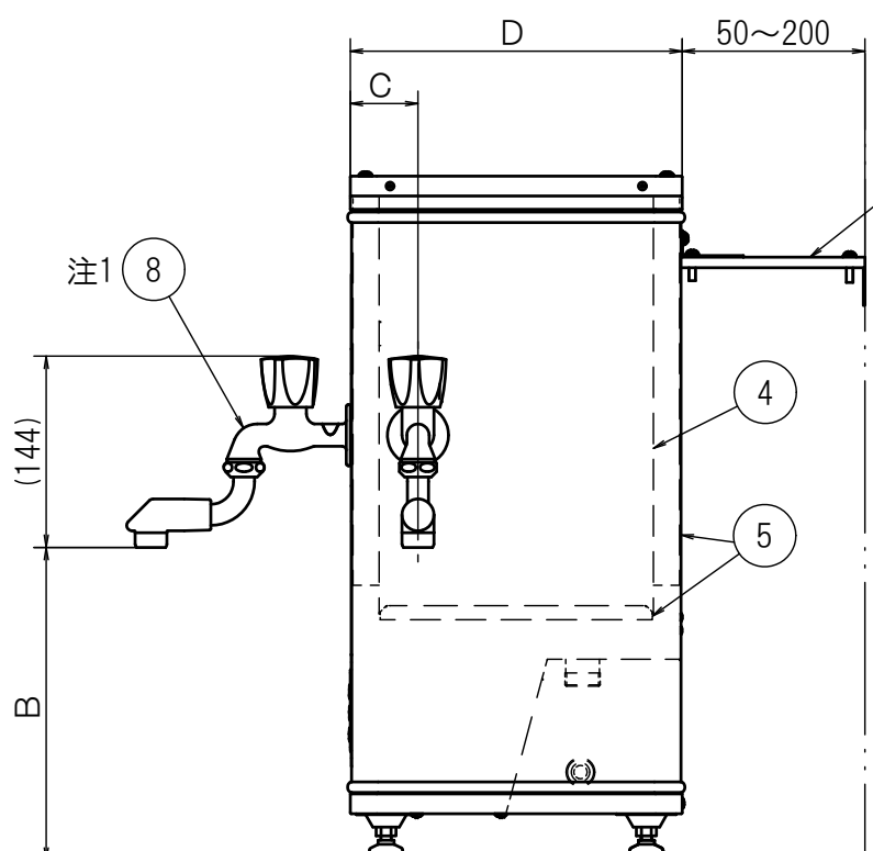
右側面図
