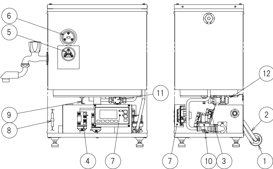
正面図
