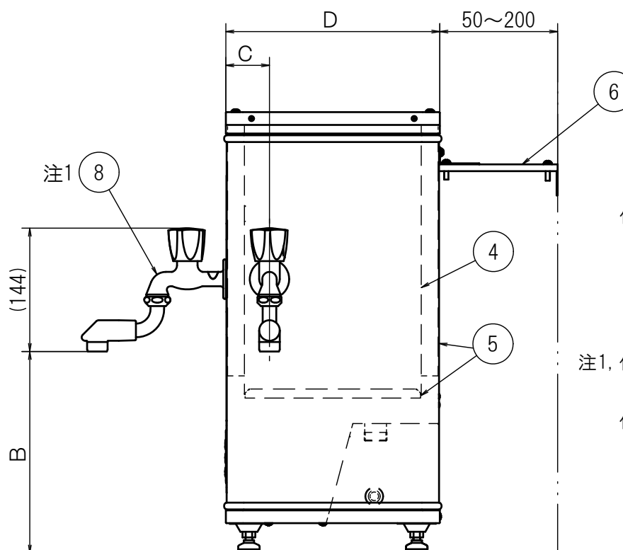
右側面図
