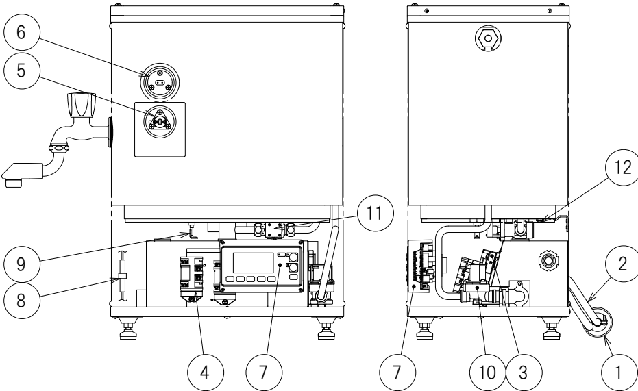
正面図
