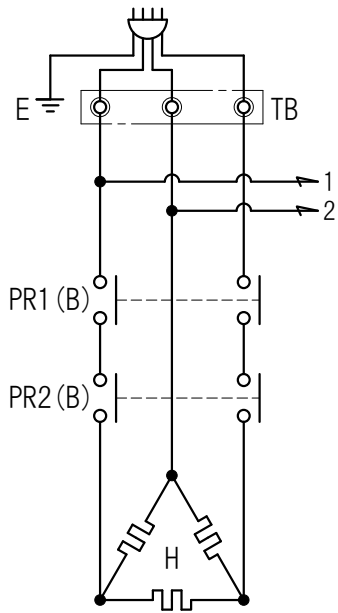
④ 三相
