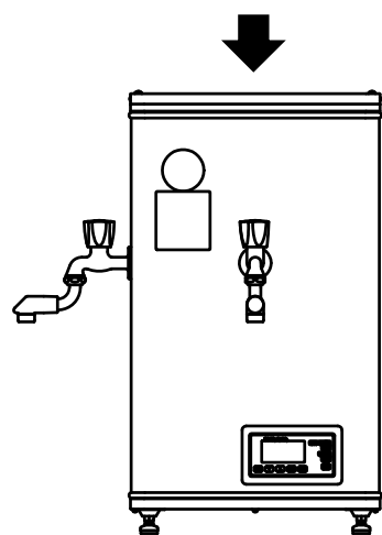
ETR□□□FL正面図
