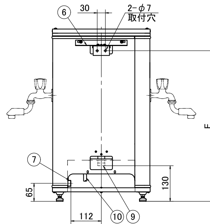
背面図
