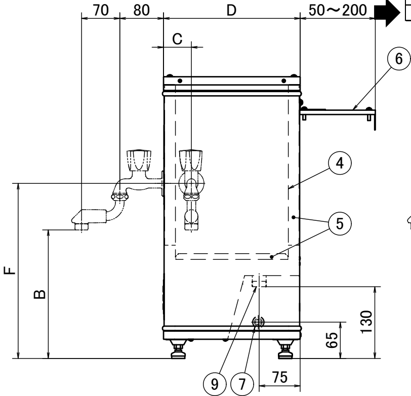
右側面図
