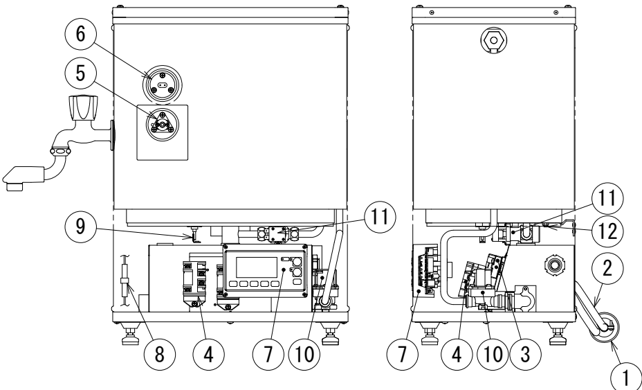
正面図
