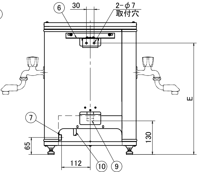
背面図
