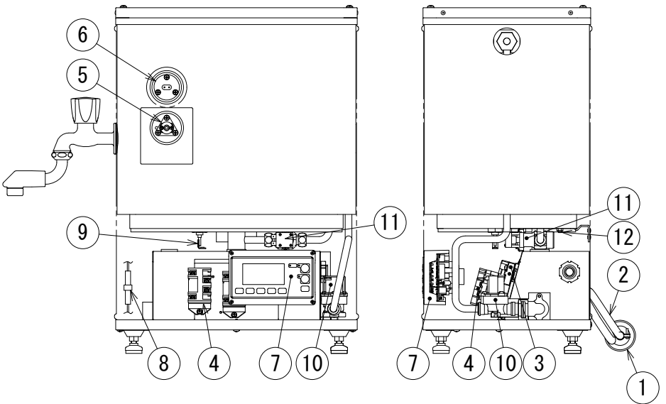
正面図
