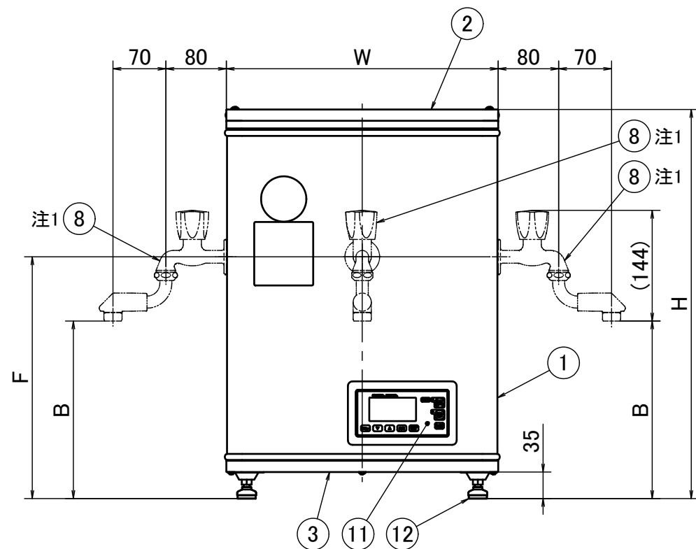
正面図
