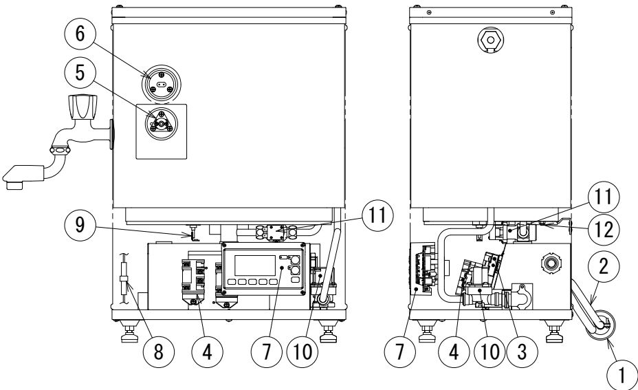
正面図
