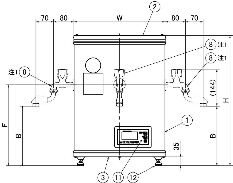
正面図
