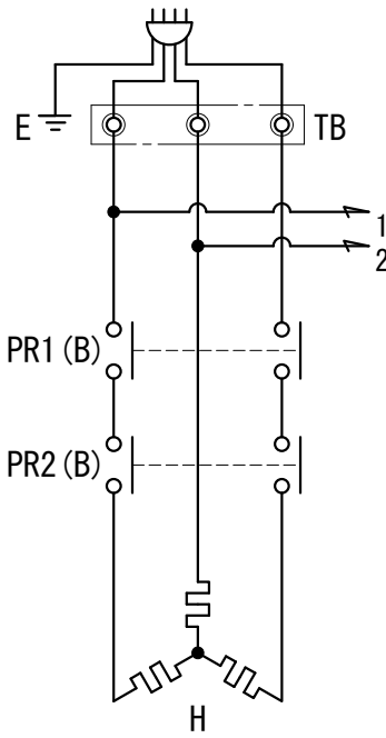
③ 三相
