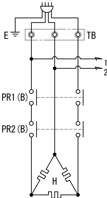
④ 三相
