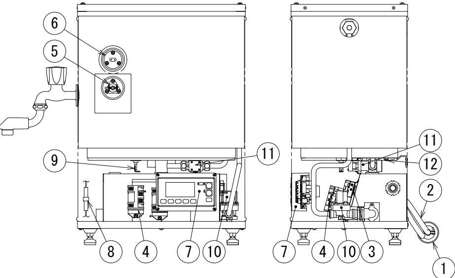
正面図
