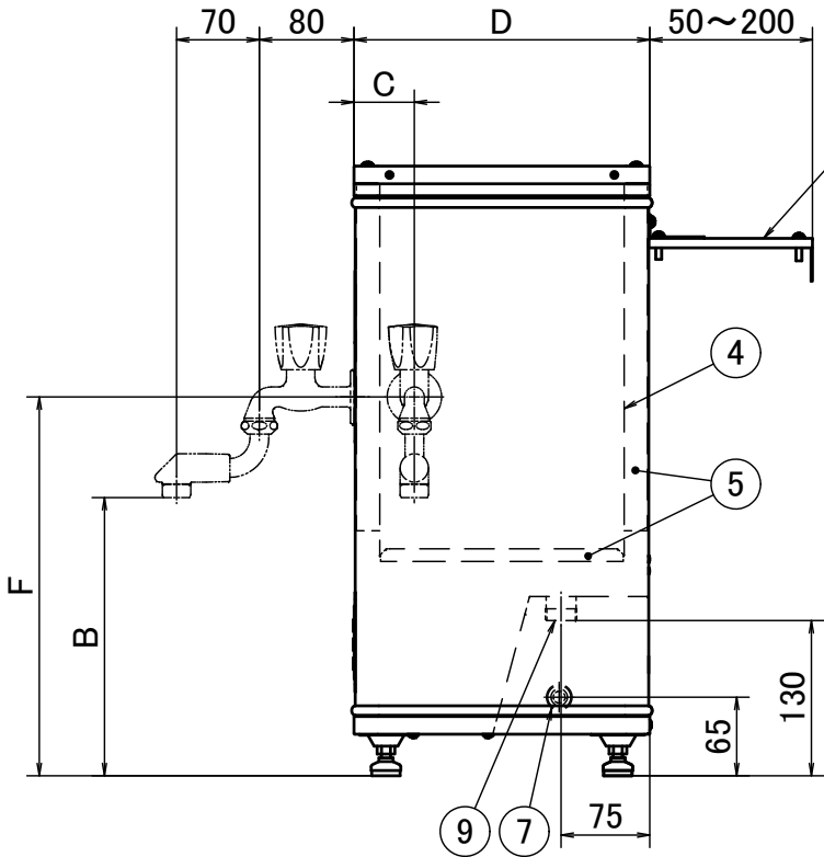
右側面図
