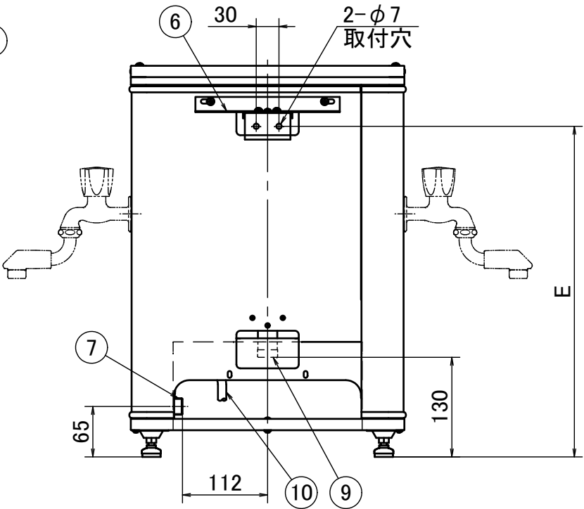
背面図
