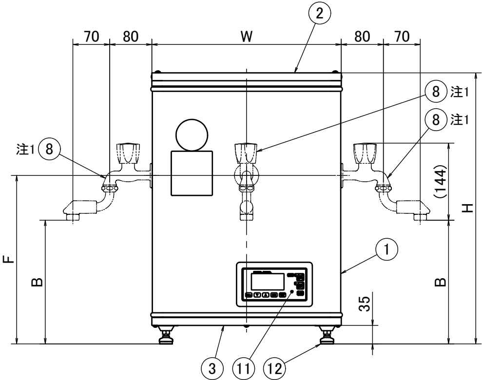
正面図
