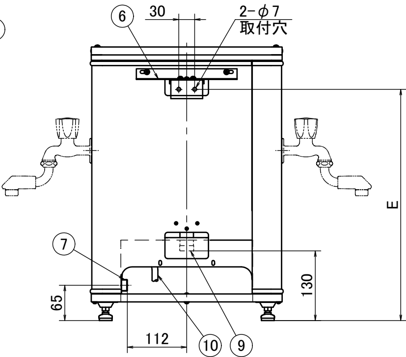
背面図
