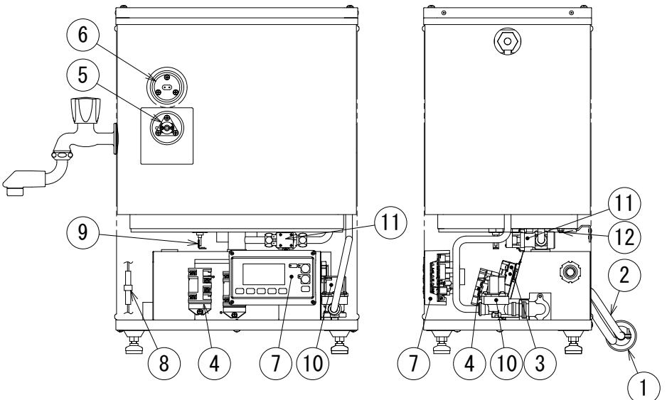
正面図
