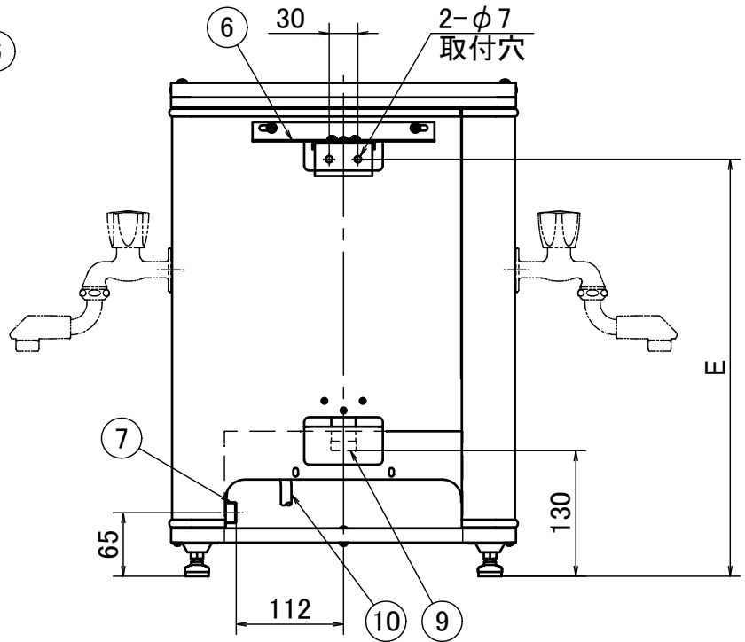
背面図
