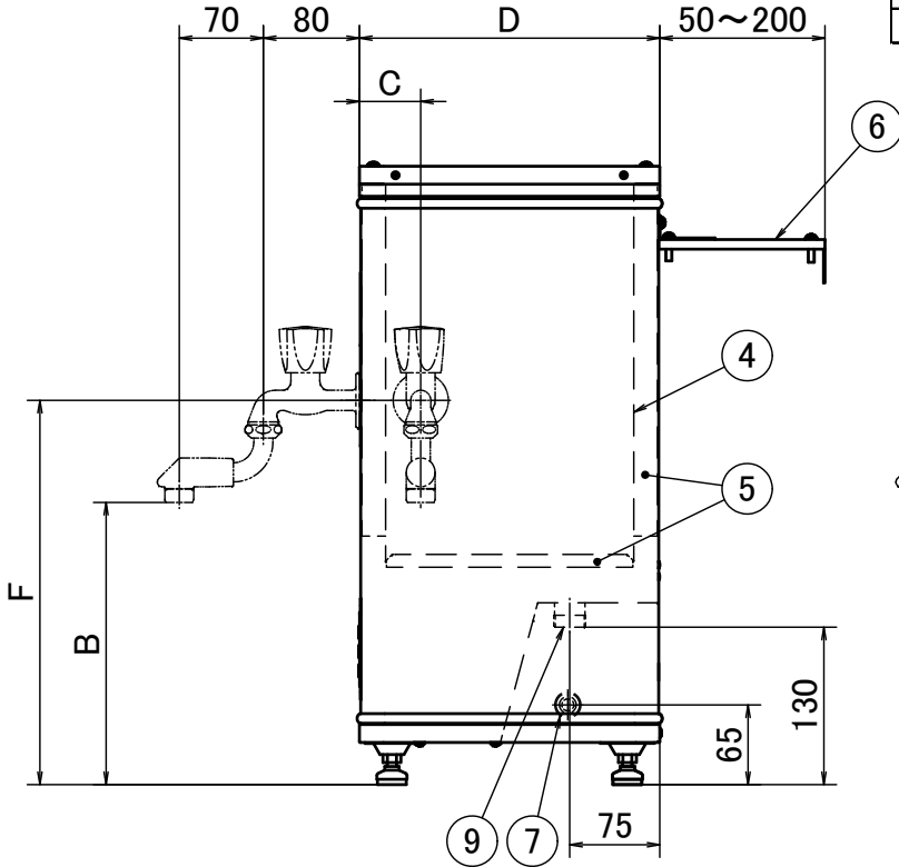
右側面図
