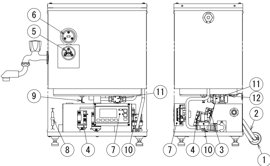
正面図
