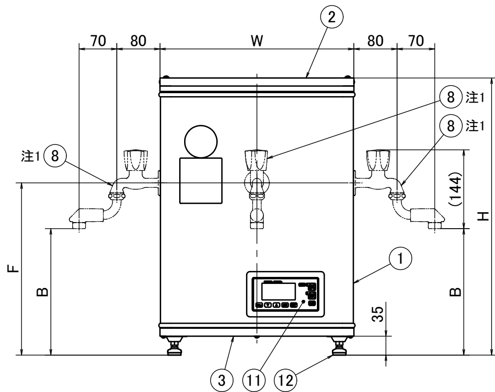
正面図
