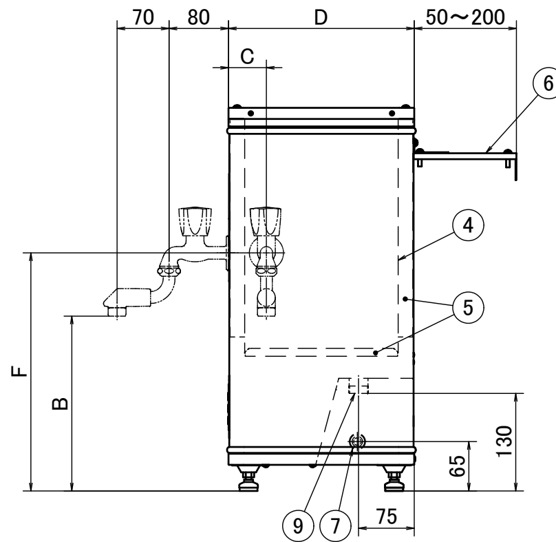
右側面図
