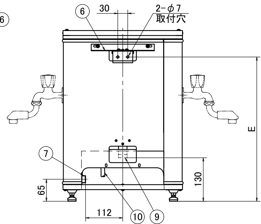
背面図
