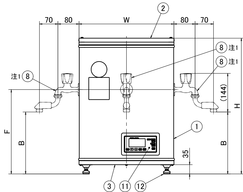
正面図
