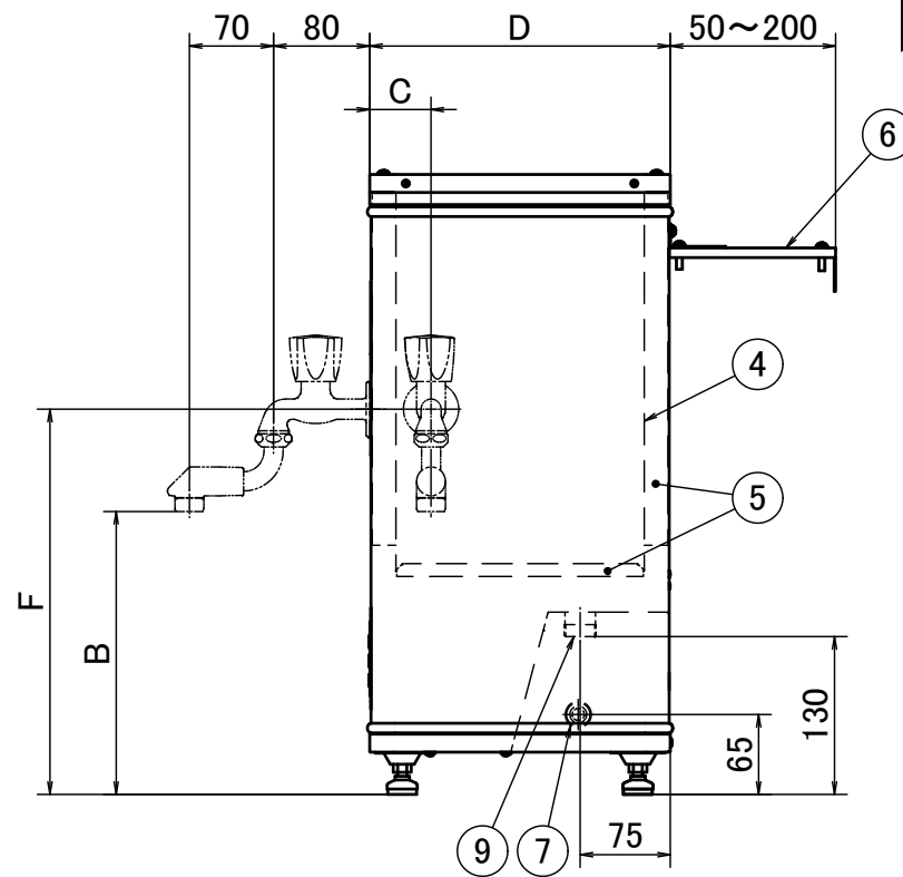
右側面図
