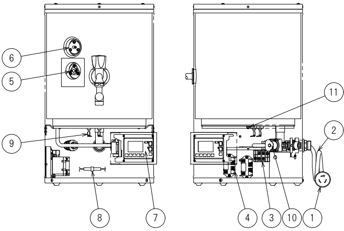
正面図
