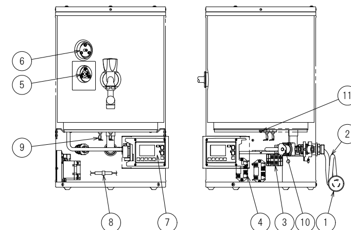
正面図
