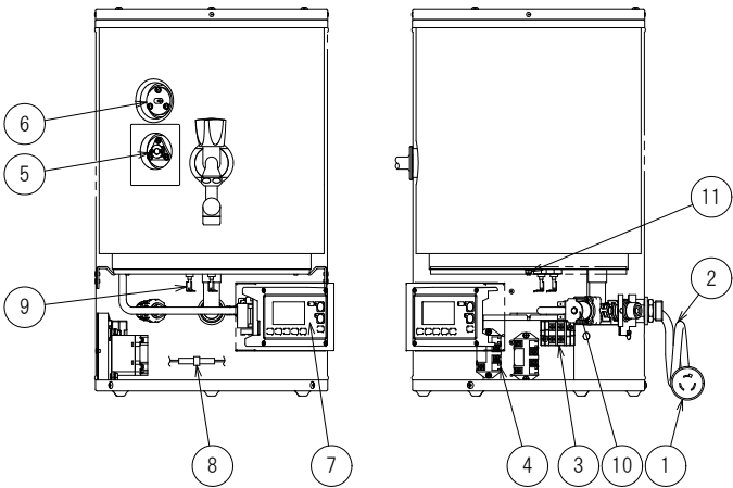
正面図 右側面図
