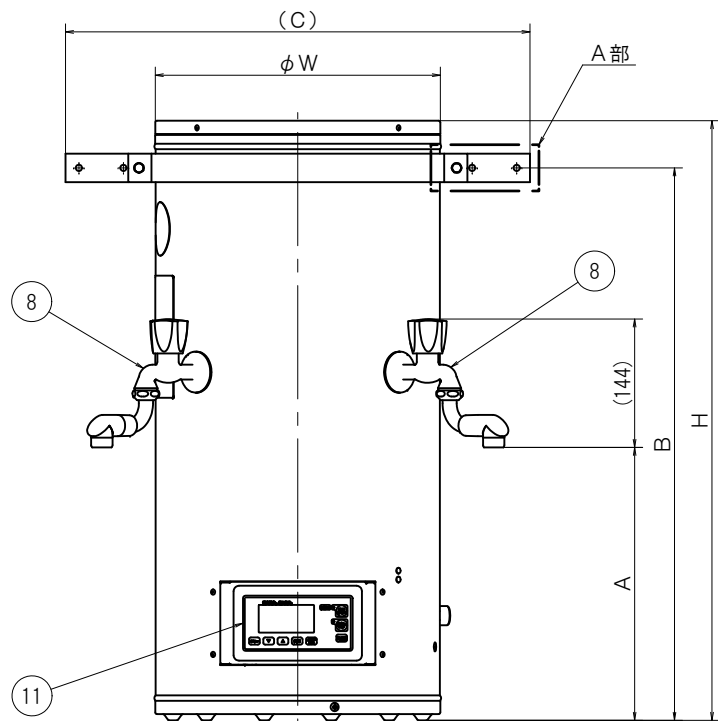
正面図
