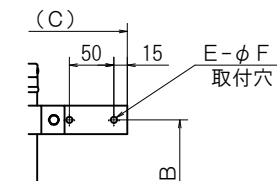
A部寸法
