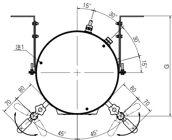
平面図
