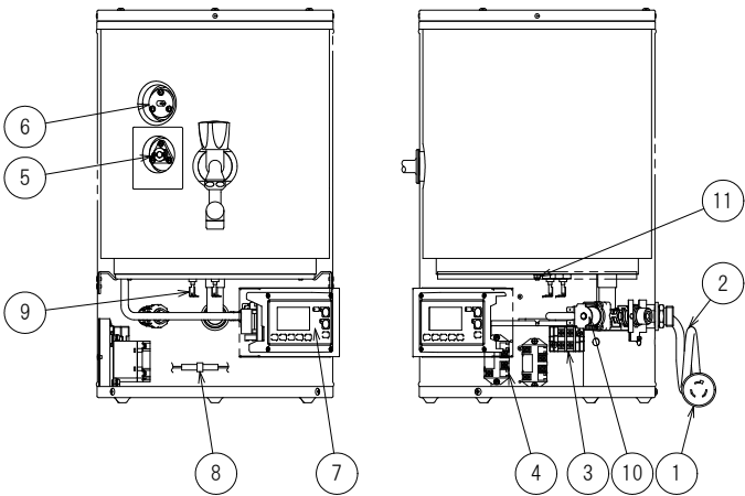
正面図
