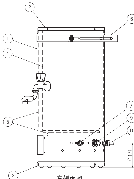
右側面図
