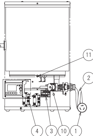
右側面図
