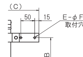
A部寸法
