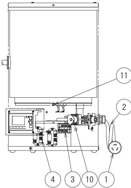
右側面図
