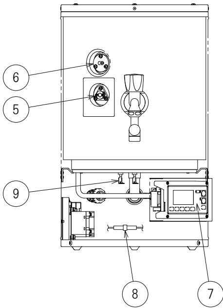
正面図
