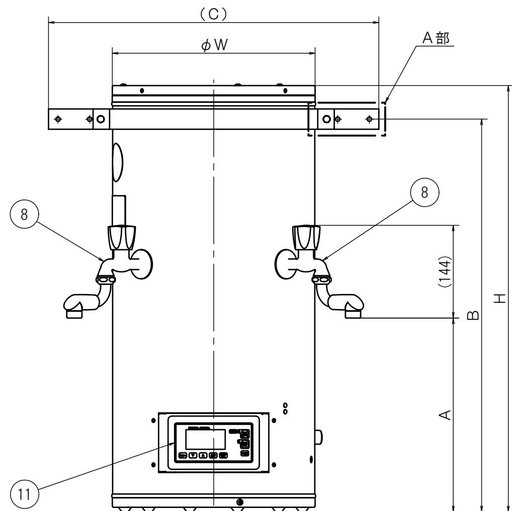
正面図
