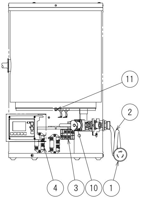
右側面図
