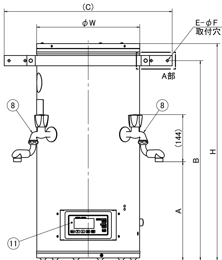
正面図
