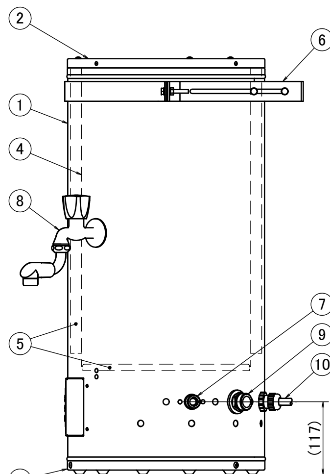
右側面図
