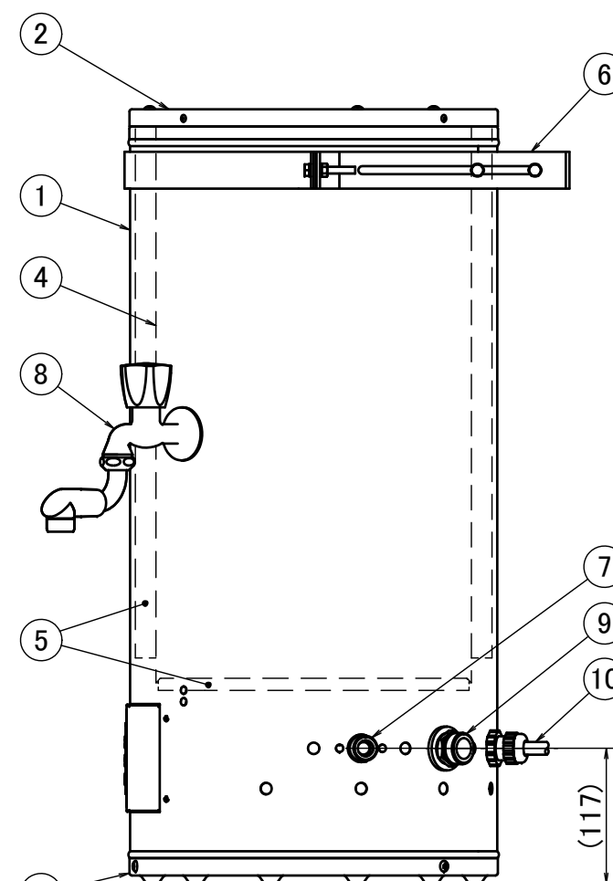
右側面図
