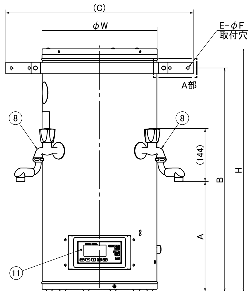
正面図
