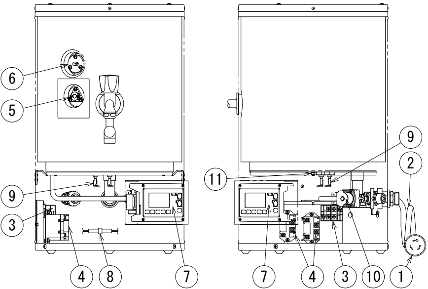
部品配置図 (図はETC12BJS)
