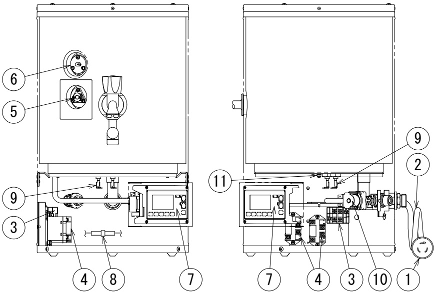
正面図
