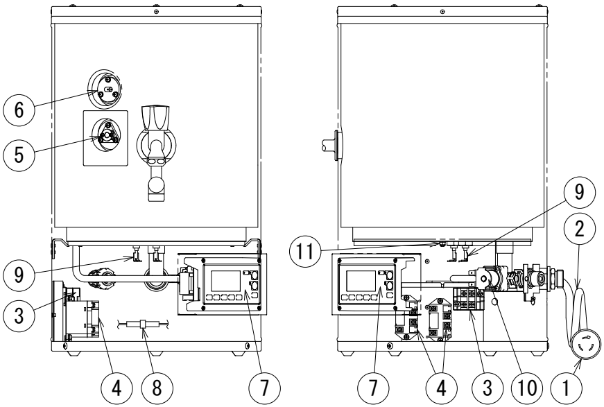
正面図
