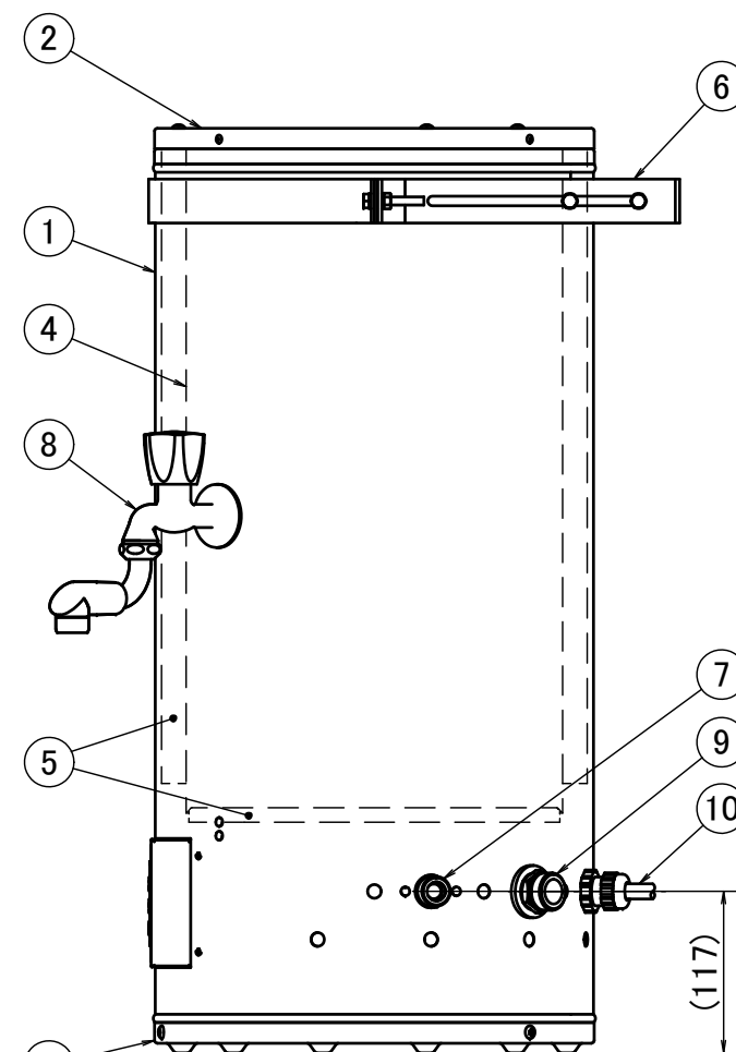
右側面図
