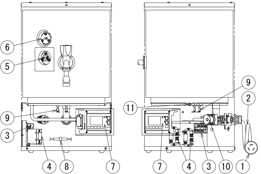
正面図
