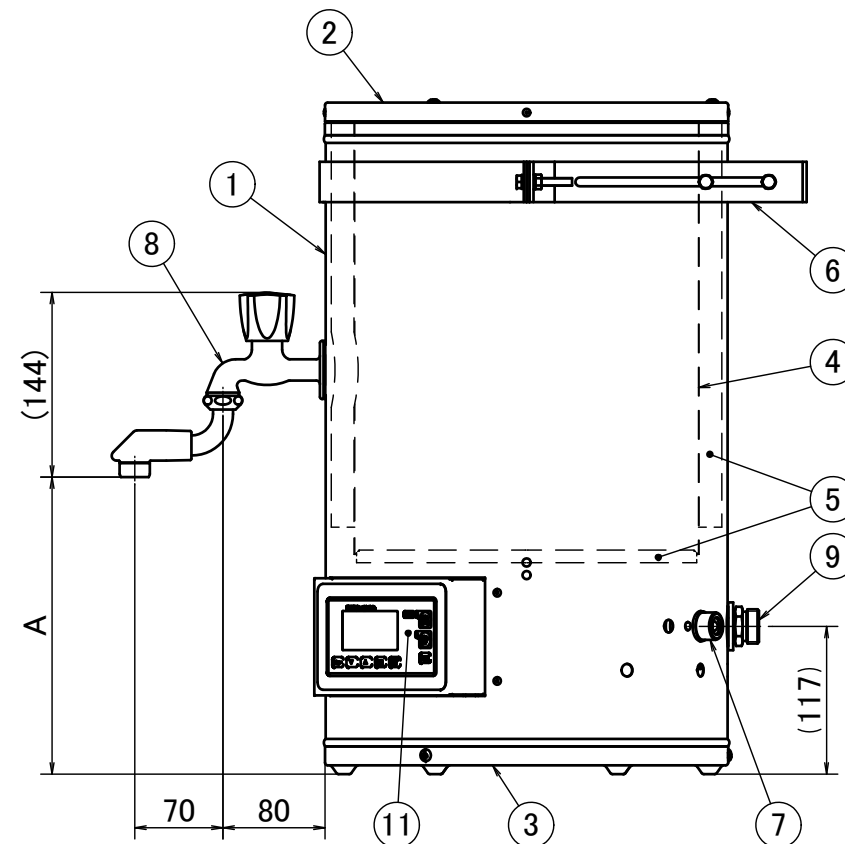
右側面図
