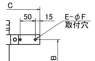
A部寸法
