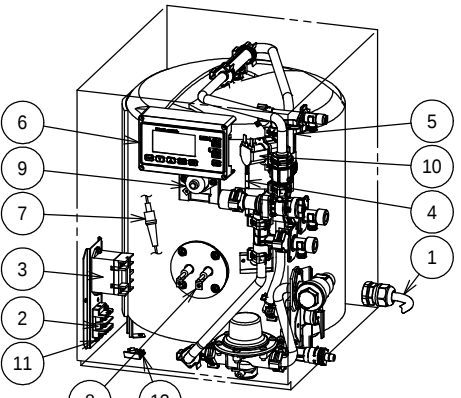
部品配置図 (図はESN20CRN)
