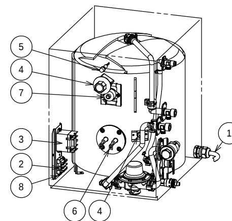
8 E アース端子 M4 — 1 7 OTH(B) 過昇温防止スイッチ 250V 20A バイメタル(リセット式) 1 OTH(A) 125V 15A, 250V 10A バイメタル(リセット式) 1 6 H ヒーター 仕様表参照 SUS316L 1 5 RL 通電表示灯 ネオンランプ(赤) — 1 4 TH 液膨式サーモスタット 30～75 — 1 3 PR(B) パワーリレー 250V 25A 2P — 1 PR(A) 250V 30A 1P — 1 2 TB(B) 電源用端子台 250V 20A 3P — 1 TB(A) 250V 20A 2P — 1 1 — 電源コード 仕様表参照 キャブタイヤケーブル 1 No 記号 名称 規格 材質・備考 数
