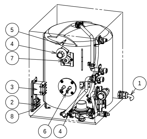
部品配置図 (図はES20ARN)
