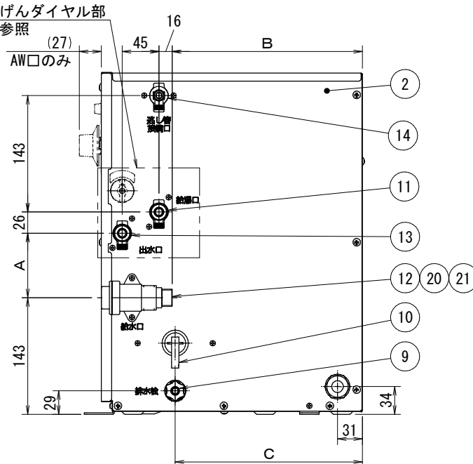
A矢視
