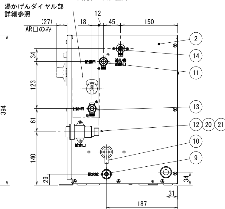
固定ねじ穴位置図
