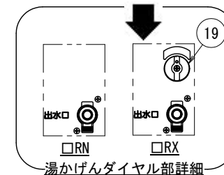
湯かげんダイヤル部詳細
