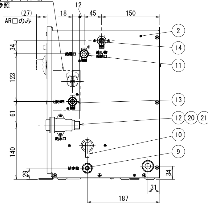
固定ねじ穴位置図
