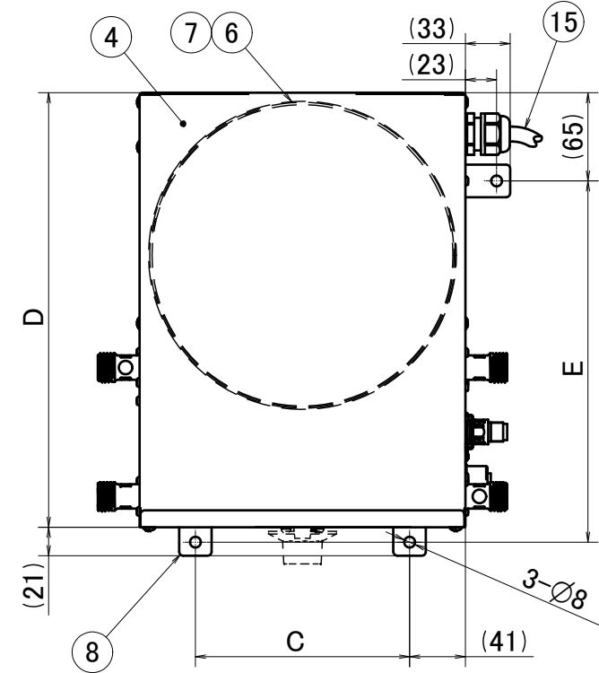
平面図
